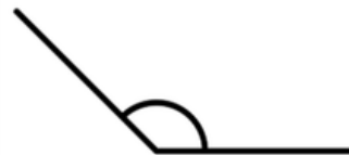
obtuse angle
