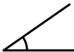
acute angle
